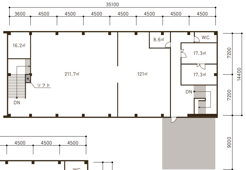
2F 平面図
