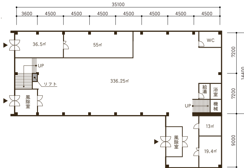
1F 平面図
