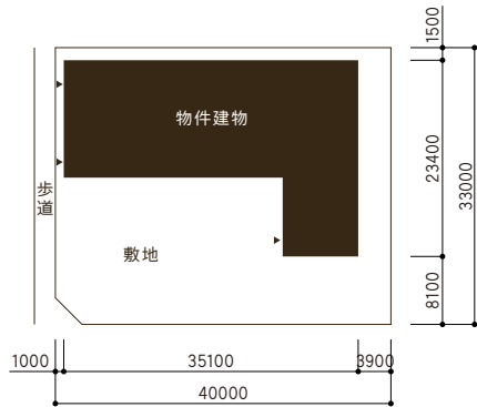
敷地平面図
