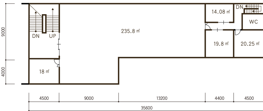
2F 平面図
