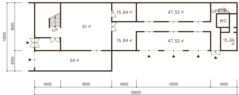
1F 平面図
